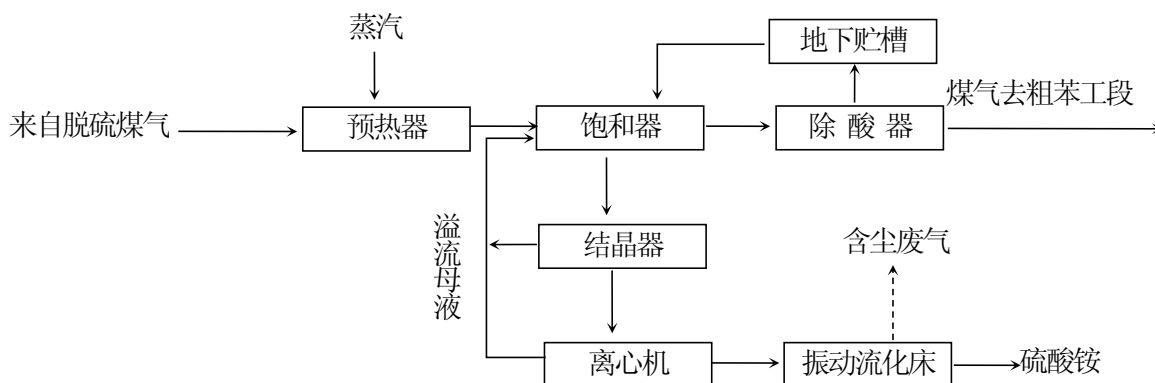
图 3.2.1-10 硫铵作业工艺流程及产污节点
