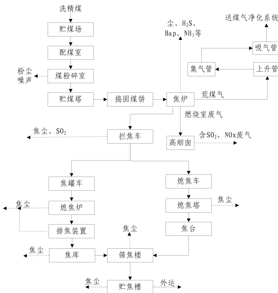
图3.2.1-6 焦化工艺流程及产污节点
