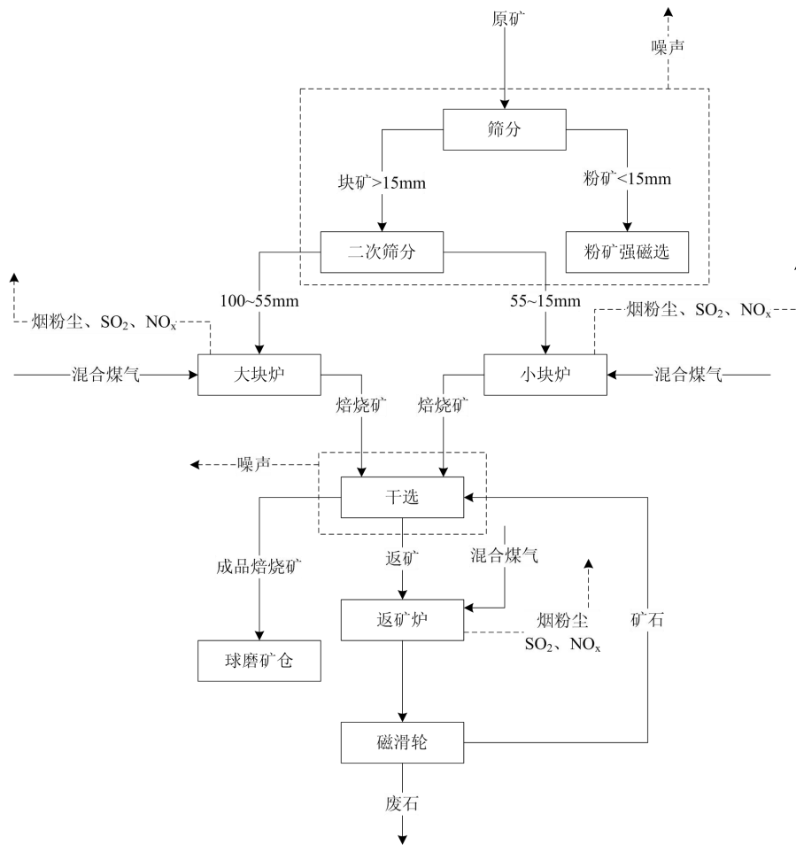
⑥ 磨选 图3.2.1-2 原矿筛分及竖炉磁化焙烧工艺流程及产污节点
