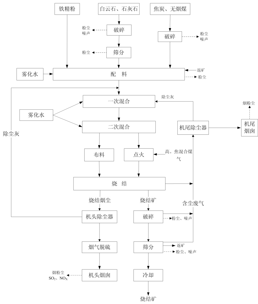
图3.2.1-5 烧结工艺流程及产污节点
